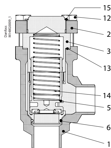
CHV-XSS 15-40
